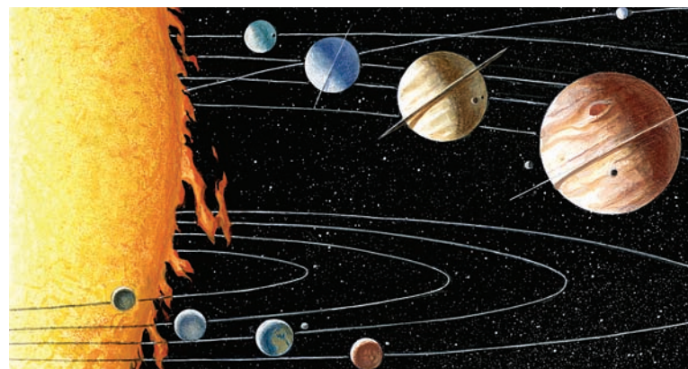
I Pianeti del Sistema Solare. La Terra (la terza da sinistra verso destra) è riconoscibile dalla Luna che le sta accanto.
