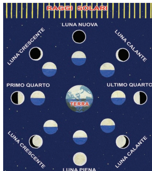
Schema delle fasi lunari: il cerchio esterno mostra la Luna vista dalla Terra; il cerchio interno mostra come la Luna è colpita dai raggi solari; al centro la Terra.
